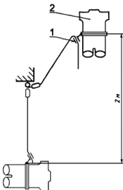
Рисунок 6 - Испытание строба статической предельной допускаемой нагрузкой
